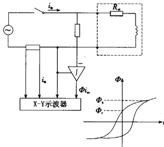
图E.0.2-2 用磁滞回环确定剩磁系数 K_r
