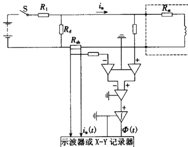
图 E.0.2-3 直流法基本电路
