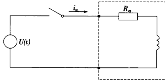
图 E.0.2-1 基本电路
