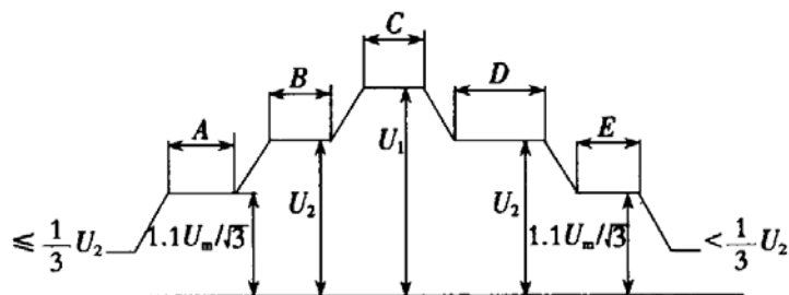
图 C.0.1 变压器长时感应电压及局部放电测量试验的加压程序
