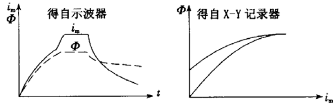
图 E.0.2-4 典型记录曲线
